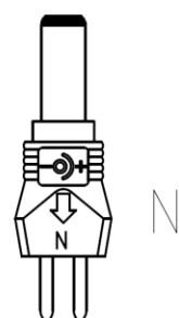
Hohlstecker/ hollowplug \varnothing 1,5 \times \varnothing 5,5 \times 12 \text{ mm}
