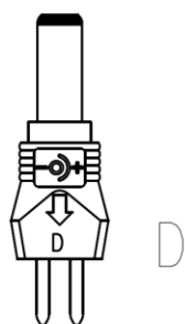
Hohlstecker/ hollowplug \varnothing 2,1 \times \varnothing 5 \times 12 \text{ mm}
