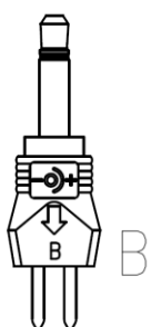
Klinkenstecker/ jackplug \varnothing 3,5 \times 15 \text{ mm}
