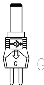
Hohlstecker/ hollowplug \varnothing 2,5 \times \varnothing 5,5 \times 12 \text{ mm}
