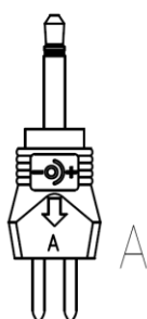
Klinkenstecker/ jackplug \varnothing 2,5 \times 13 \pm 0,5 \text{ mm}
