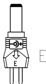
Hohlstecker/ hollowplug \varnothing 2,1 \times \varnothing 5,5 \times 12 \text{ mm}
