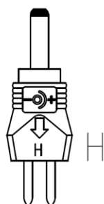
Hohlstecker/ hollowplug \varnothing 1,35 \times \varnothing 3,5 \times 10 \text{ mm}
